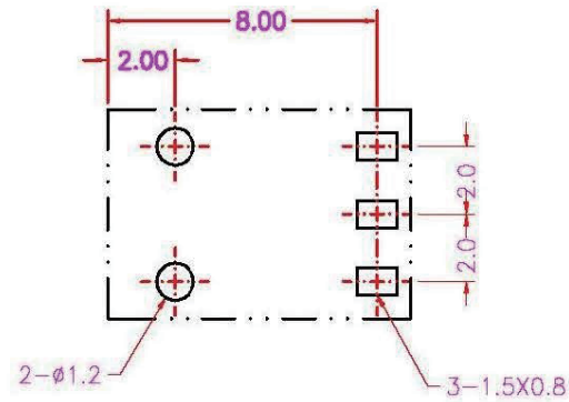
印制板开孔示意图
